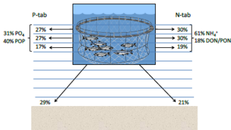
Figur 4. Fordeling af N- og P-tab fra havbrug til det omgivende miljø i den økologiske model(DHI)
