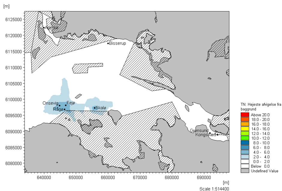
Figur 6. Den maksimale virkning på baggrundskoncentrationen af TN (%) pga. NH 4 -udledninger fra Skalø, Fejø, Rågø og Onsevig havbrug. Skraverede områder er Natura 2000 områder.
