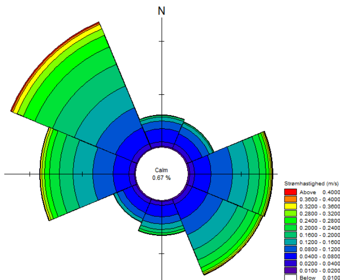
Figur 1 Modelleret årlig overfladestrøm (2 meter) i 2005 ved Skalø Havbrug.
