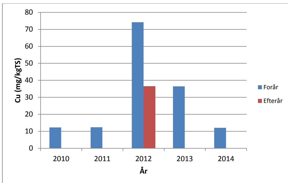
Figur 7: Analyser af kobber i bundsediment fra den samlede prøvetagning på 5 lokaliteter under Skalø Havbrug (2010-2014). En ekstra prøve blev analyseret om efteråret 2012.
