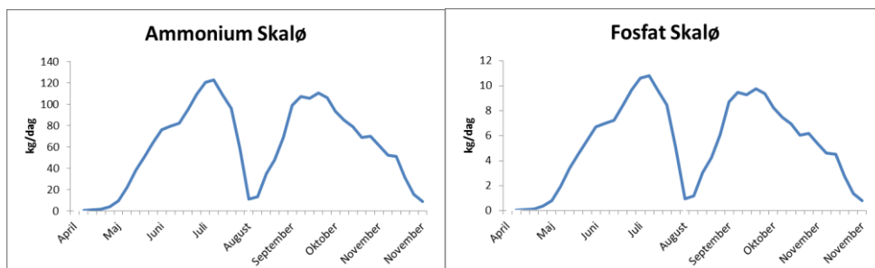
Figur 5. Udviklingen i udledningen af \text{NH}_4^+ samt fosfat i løbet af produktionssæsonen (april-november) ved Skalø havbrug.
